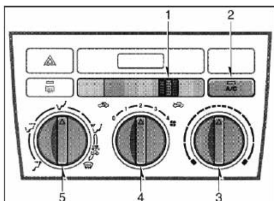
手动空调控制面板
